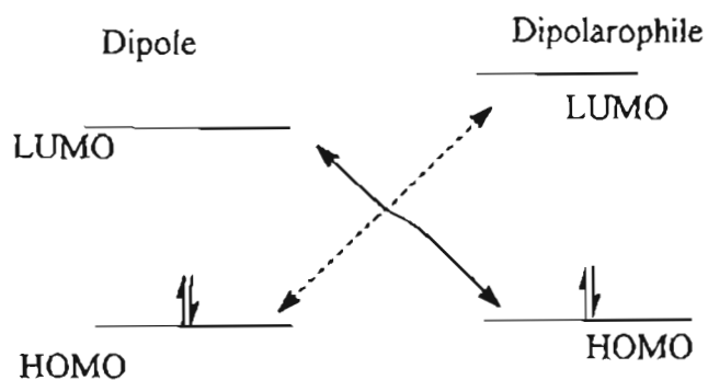
Type 3 (LUMO Controlled)
